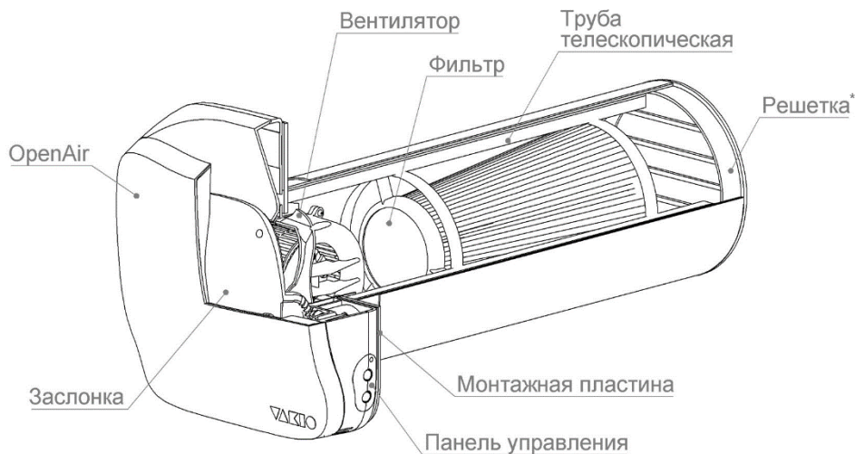
Рис. 1 Общий вид прибора. *Вариант с металлической решёткой.
