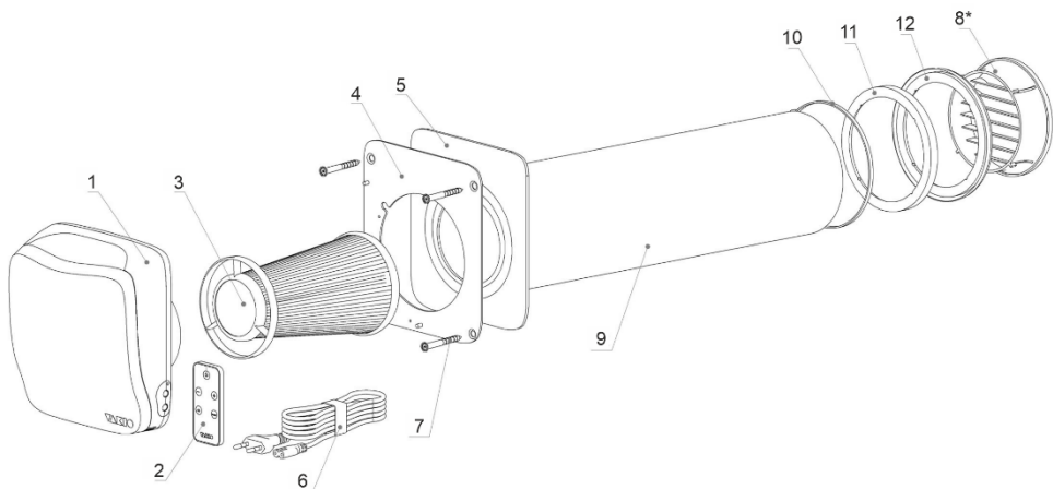
Рис. 2 Состав комплекта поставки. *Вариант с пластиковой решеткой.
