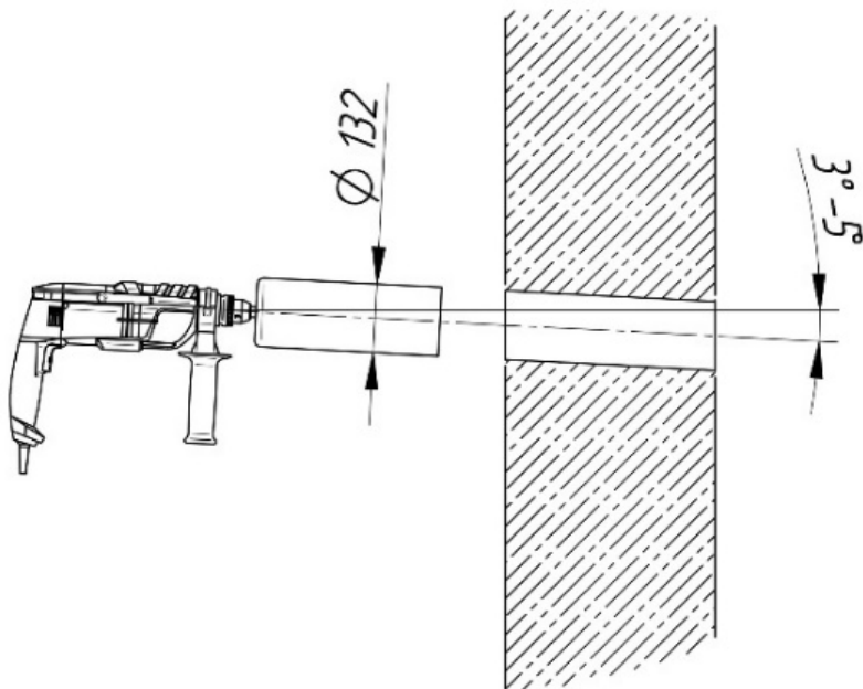
Рис. 3 Бурение отверстия
