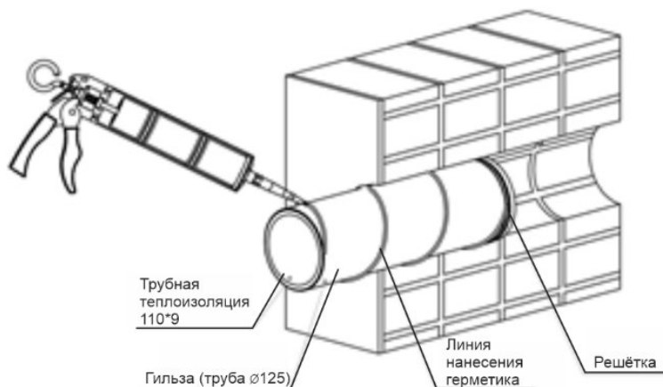
Рис. 4 Вариант установки гильзы с нанесением герметика
